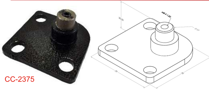
Recibidor rodamiento 6203
