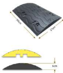
8166 Reductores de velocidad
