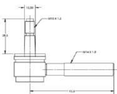
Rótula articulación de puertas de servicio de autobuses M14 x 1.5
